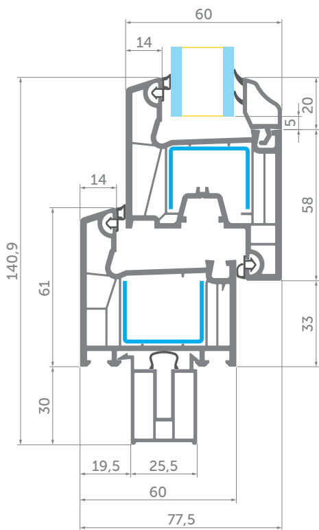
Вікно з однією стулкою
